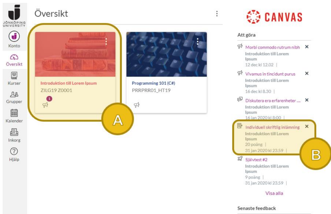
Figur 1: Canvas översikt.
